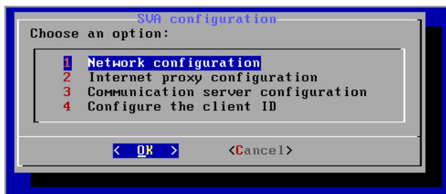
Interfaz de configuración del Security Server (menú principal)
